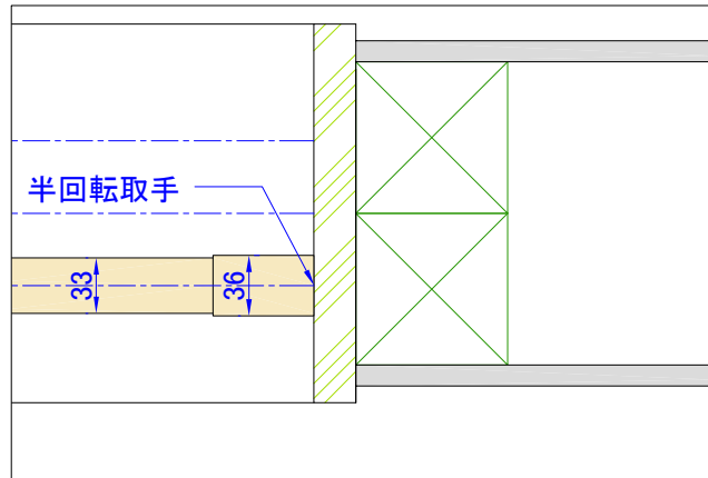
右端部断面詳細図 S=1:5
