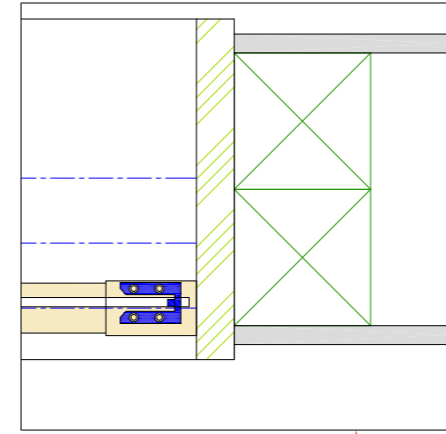
右端部断面詳細図 S=1:5
