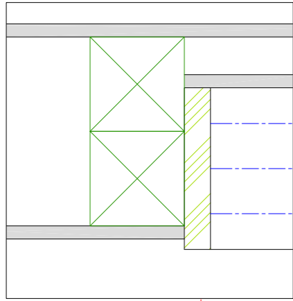
左端部断面詳細図 S=1:5
