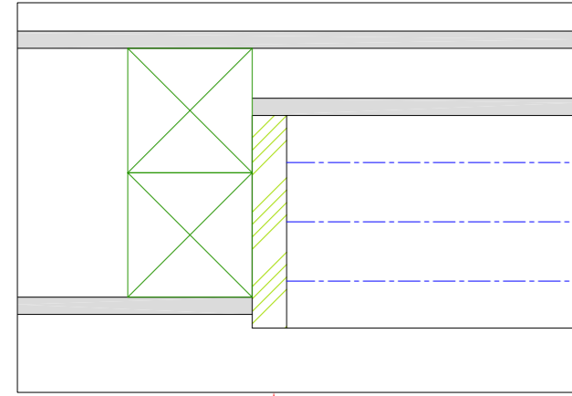
左端部断面詳細図 S=1:5
