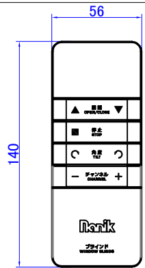
防水型5チャンネルRFリモコン姿図
